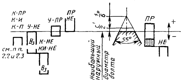
Калибры для контроля болтов (наружной резьбы)
