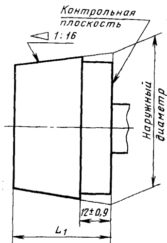
Калибр-пробка Г
